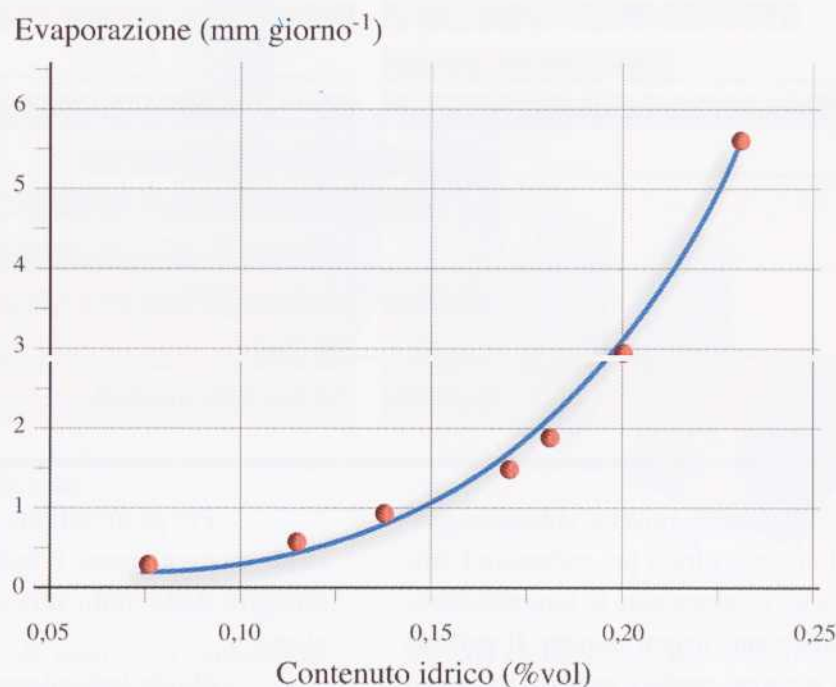
FIGURA 4 - RELAZIONE TRA EVAPORAZIONE E CONTENUTO IDRICO DEL SUOLO, RILEVATO NEI PRIMI 8 cm DI PROFONDITÀ. I DATI SI RIFERISCONO AD UN OLIVETO ADULTO CON SESTO D'IMPIANTO 7x7 m E CON ETO GIORNALIERO PARI A 8 mm (DA FERNÁNDEZ. & MORENO, 1999)
