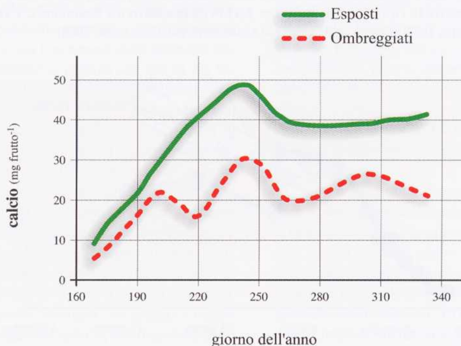
FIGURA 7 - CONTENUTO DI CALCIO IN FRUTTI DI ACTINIDIA SOTTOPOSTI A DIVERSO REGIME RADIATIVO (DA MONTANARO, 2001)
