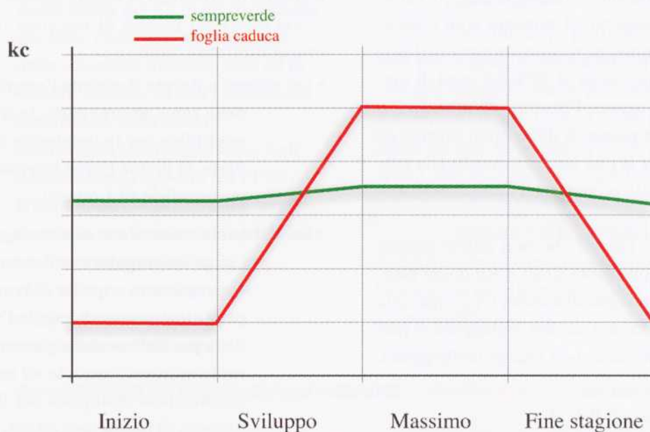
FIGURA 3 - ANDAMENTO DEL K_c IN PIANTE A FOGLIA CADUCA E SEMPREVERDI DURANTE LE VARIE FASI DELLA STAGIONE VEGETATIVA (FAO, 1998)
