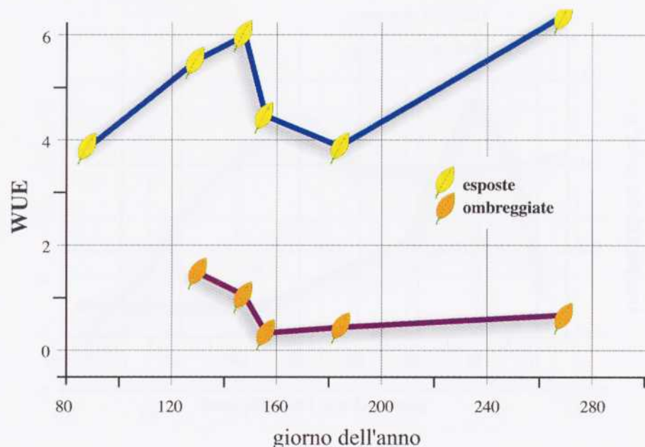
FIGURA 10 - WUE IN FOGLIE ESPOSTE (GIALLE) ED OMBREGGiate (MARRONI) DI ALBICOCCO IN PIENA PRODUZIONE DURANTE IL CICLO ANNUALE (DA XILOYANNIS ET AL., 1999b)
