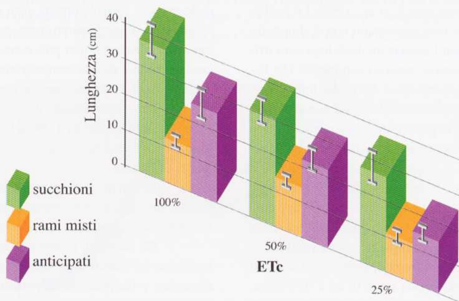
FIGURA 5 - CRESCITA IN DIVERSI TIPI DI RAMO REGISTRATA DA FINE GIUGNO ALL'INIZIO DI OTTOBRE, IN PIANTE DI PESCO SOTTOPOSTE A DIVERSI REGIMI IDRICI (DA DICHIO ET AL., 2001)
